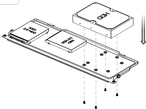
SSD / 2.5" HDD
